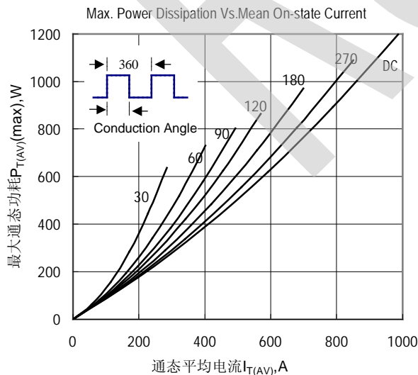
Fig.5 大功耗与平均电流关系曲线
