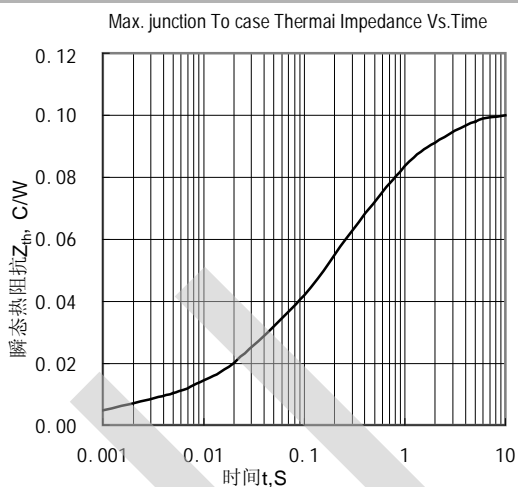
Fig.2 结至管壳瞬态热阻抗曲线
